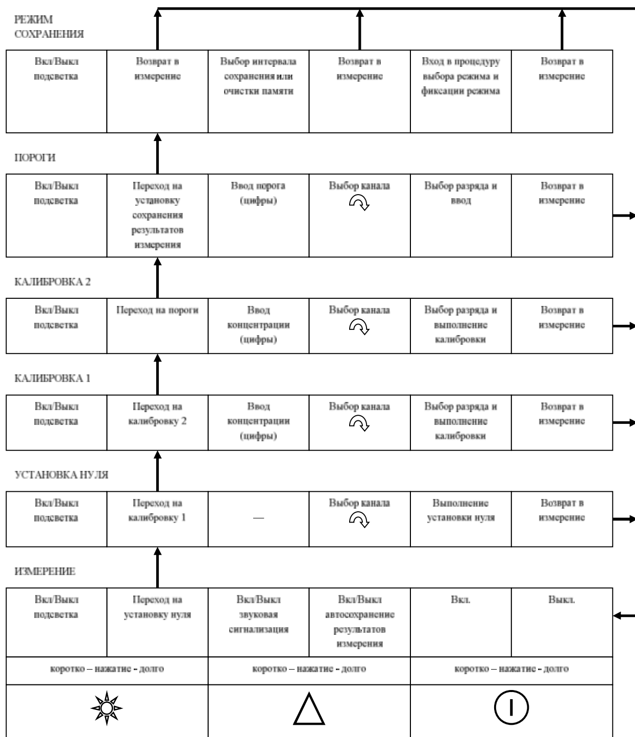
Рисунок 1. Алгоритм выбора режимов работы газоанализатора
