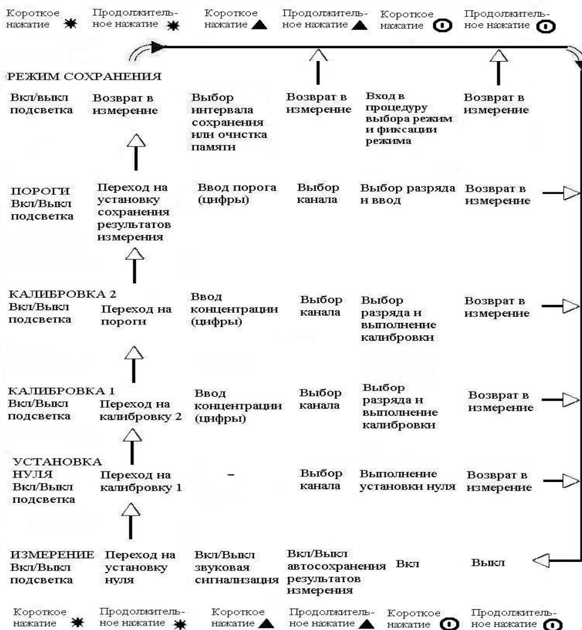
Рисунок 1 – Диаграмма выбора режимов работы газоанализатора
